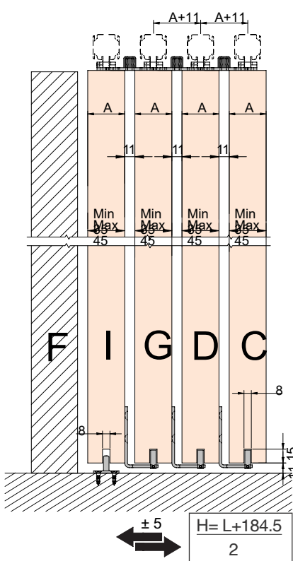
4 HOJAS TELESCÓPICAS / 4 PANEL
