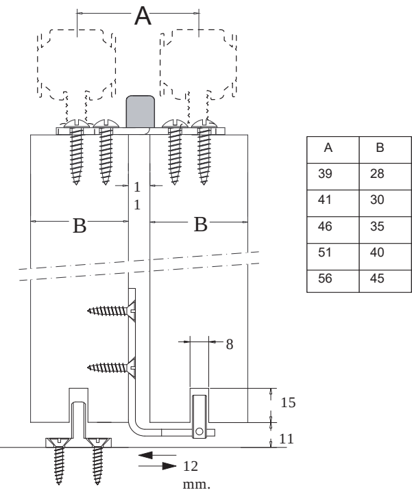
2 HOJAS TELESCÓPICAS / 2 PANEL
