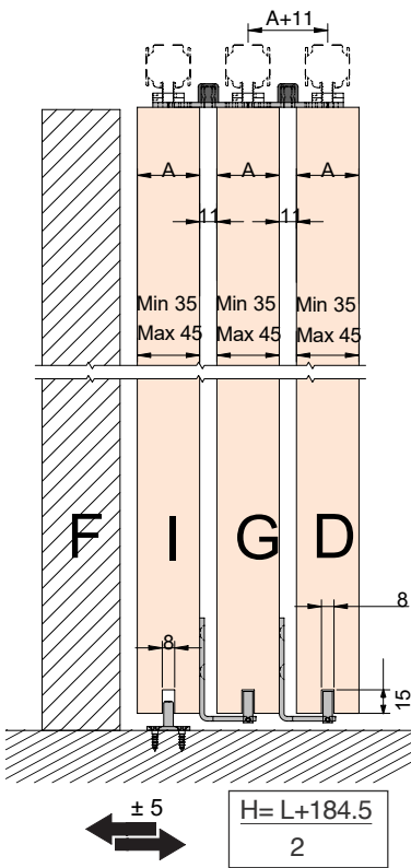
3 HOJAS TELESCÓPICAS / 3 PANEL
