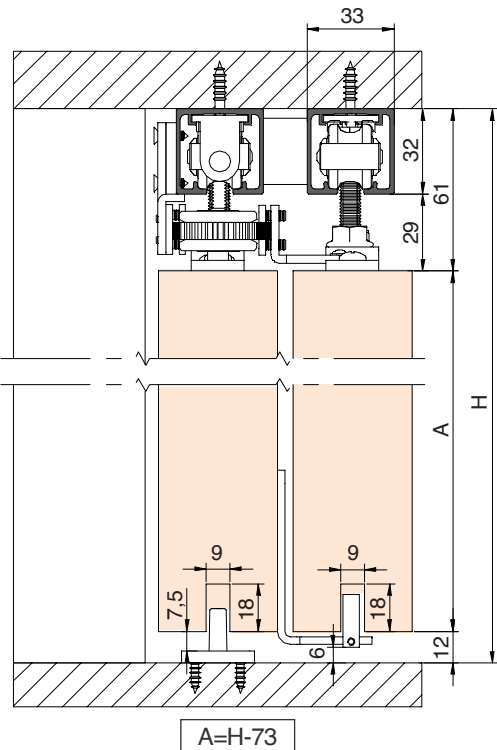
SF-TELESCÓPICA PROGRESIVA 2 HOJAS | PANELS
