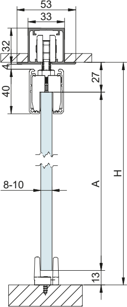
STAR FT VIDRIO FIJO | FIXED GLASS | VERRE FIXE
