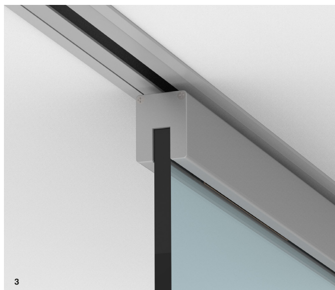
A Perfil funda FT | Support FT track | Rail de couverture FT. B Perfil Star | Star track | Rail Star. C Diseño de perfil con avellanado integrado | Track design with drilled countersink | Conception de rail avec fraisage intégré.
