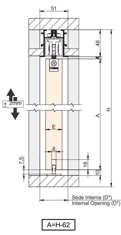
MONTAJE FALSO TECHO /False Ceiling Mount
