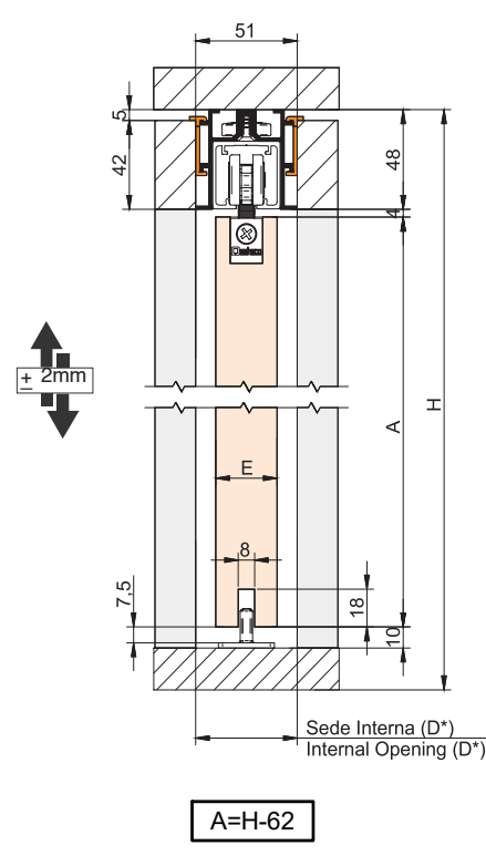
MONTAJE PERFIL VISTO /Ceiling mount
