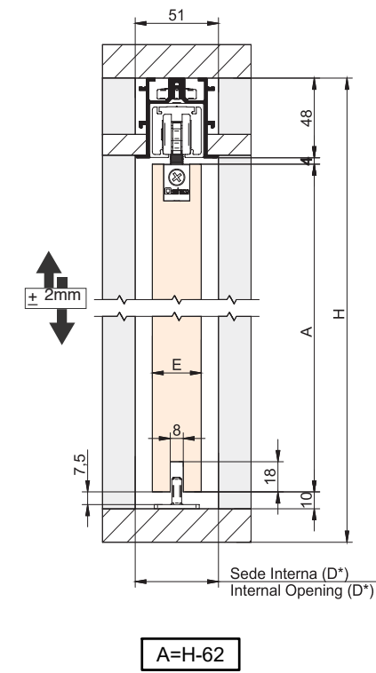
MONTAJE FALSO TECHO /False Ceiling Mount
