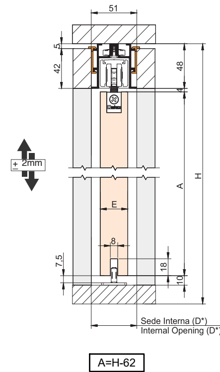
MONTAJE PERFIL VISTO /Ceiling mount
