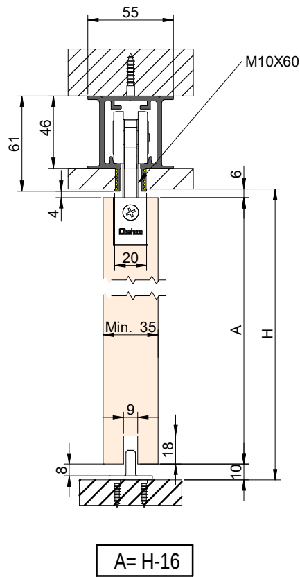
PERFIL STAR FTI XL FALSO TECHO INVISIBLE Star Track FTI XL False Ceiling Invisible
