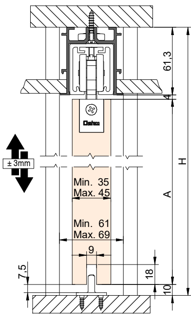
MONTAJE FALSO TECHO /False Ceiling Mount
