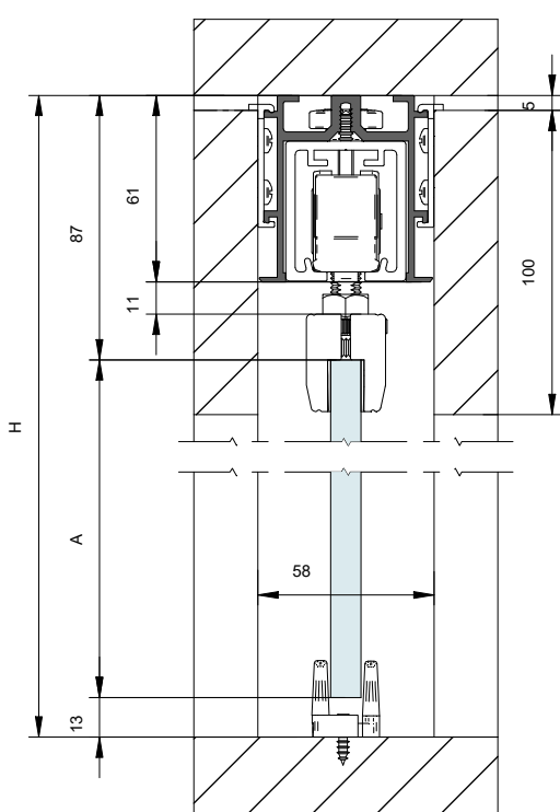
MONTAJE PERFIL VISTO /Ceiling mount
