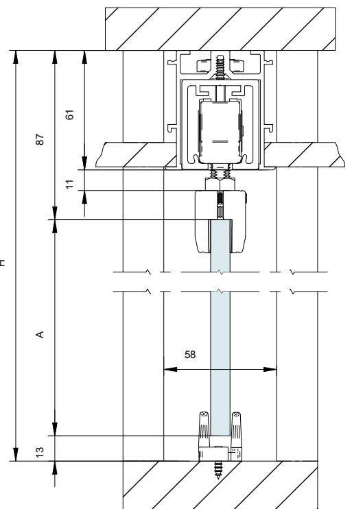
MONTAJE FALSO TECHO /False Ceiling Mount
